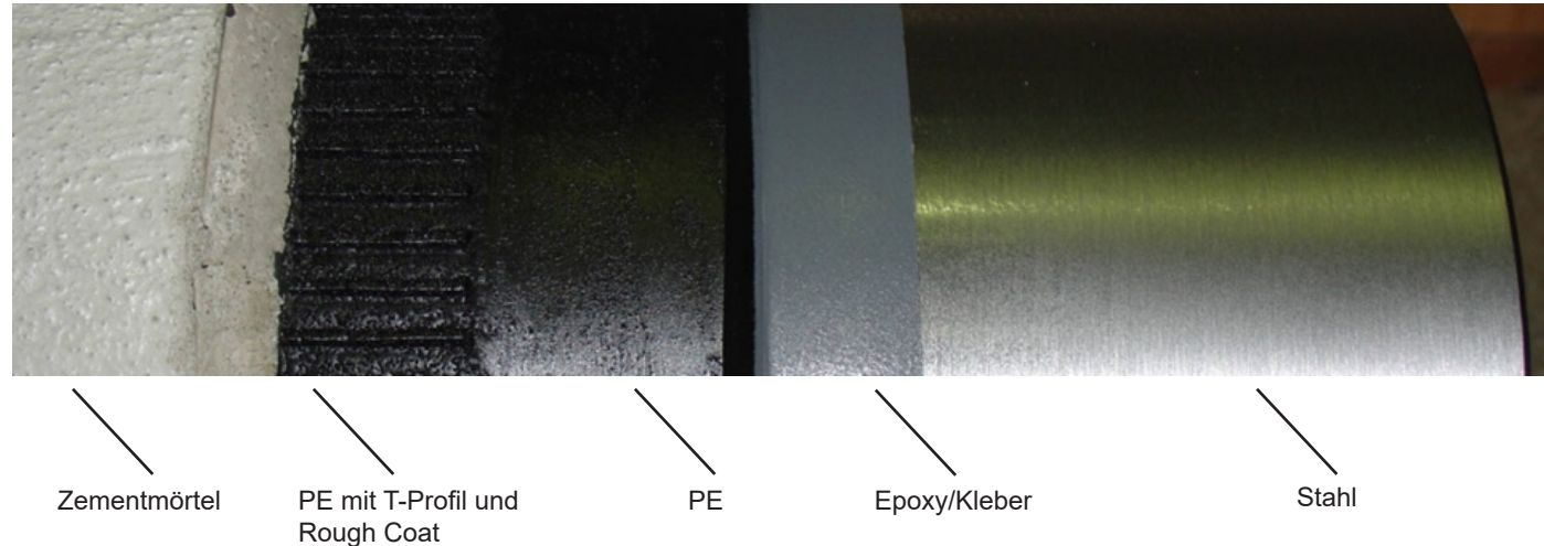
Abbildung 7: Endenausführung der FZM-S-Ausführung
