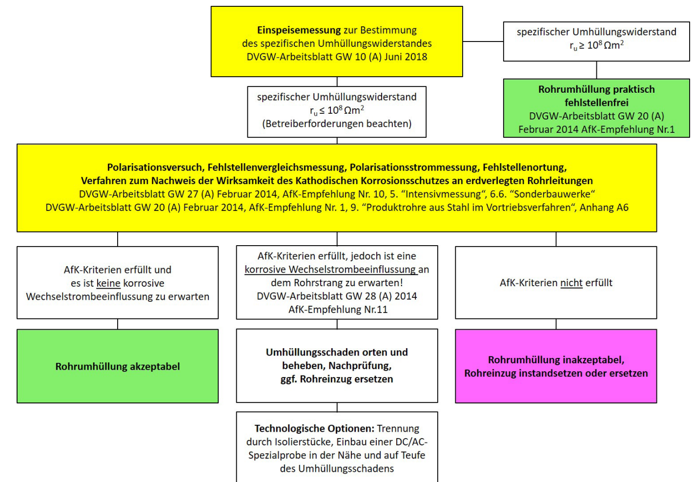
Abbildung 2: Umhüllungsprüfung an grabenlos verlegten Stahlrohrleitungen
